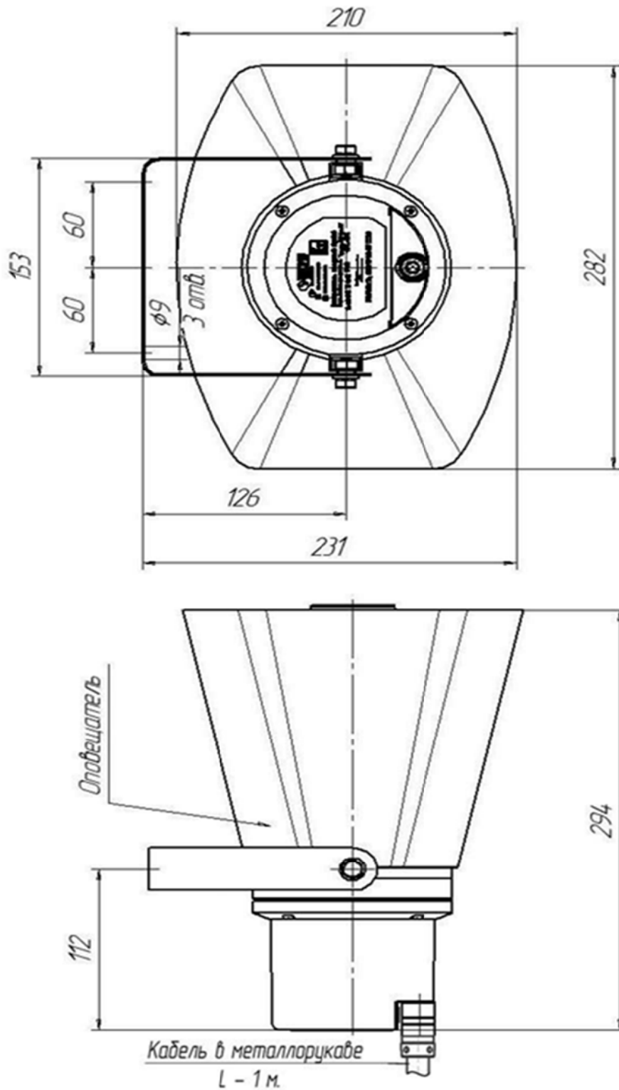
Рисунок 1 – габаритные размеры оповещателя
